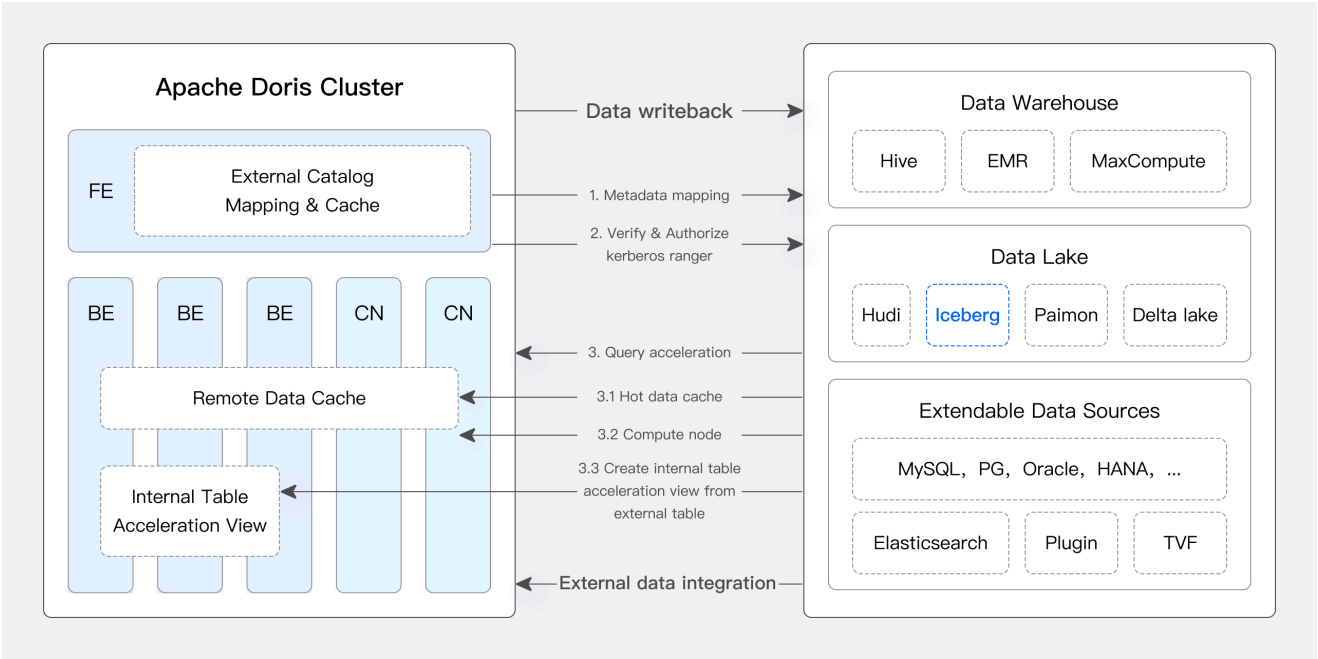
使用 Doris 和 Iceberg 构建 Lakehouse
