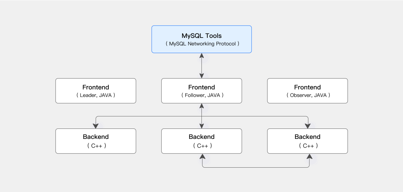
存算一体架构
