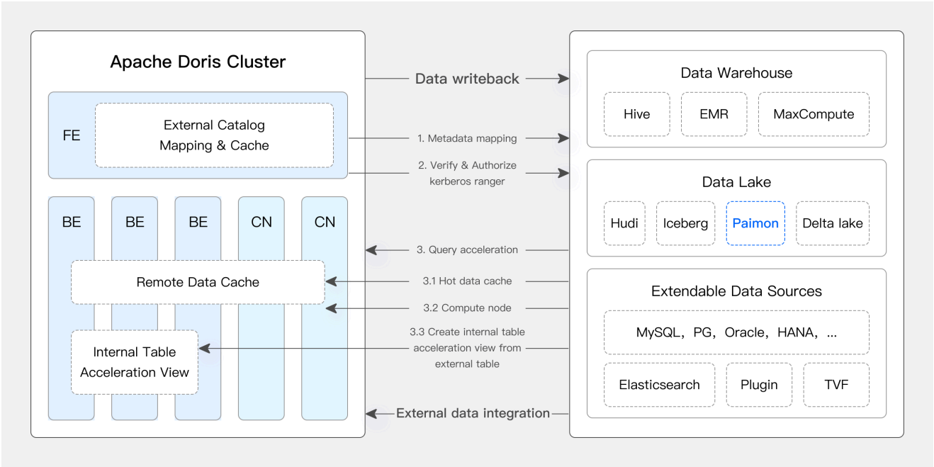
使用 Doris 和 Paimon 构建 Lakehouse
