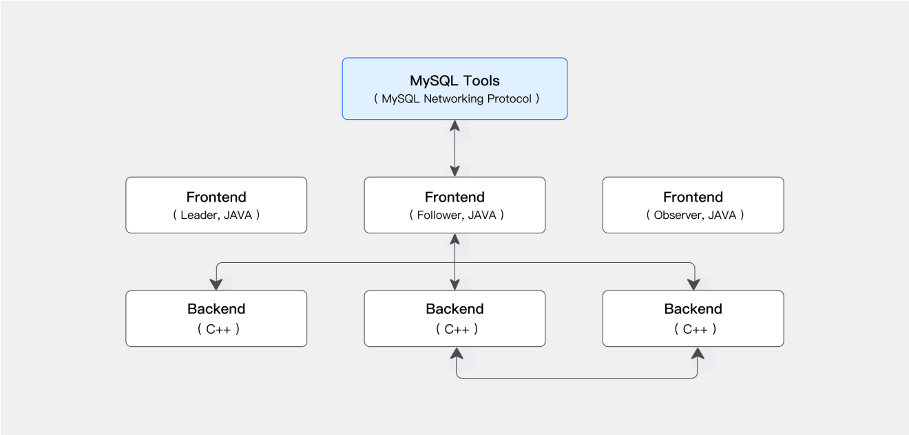
MPP 数据库整体架构和技术特点
