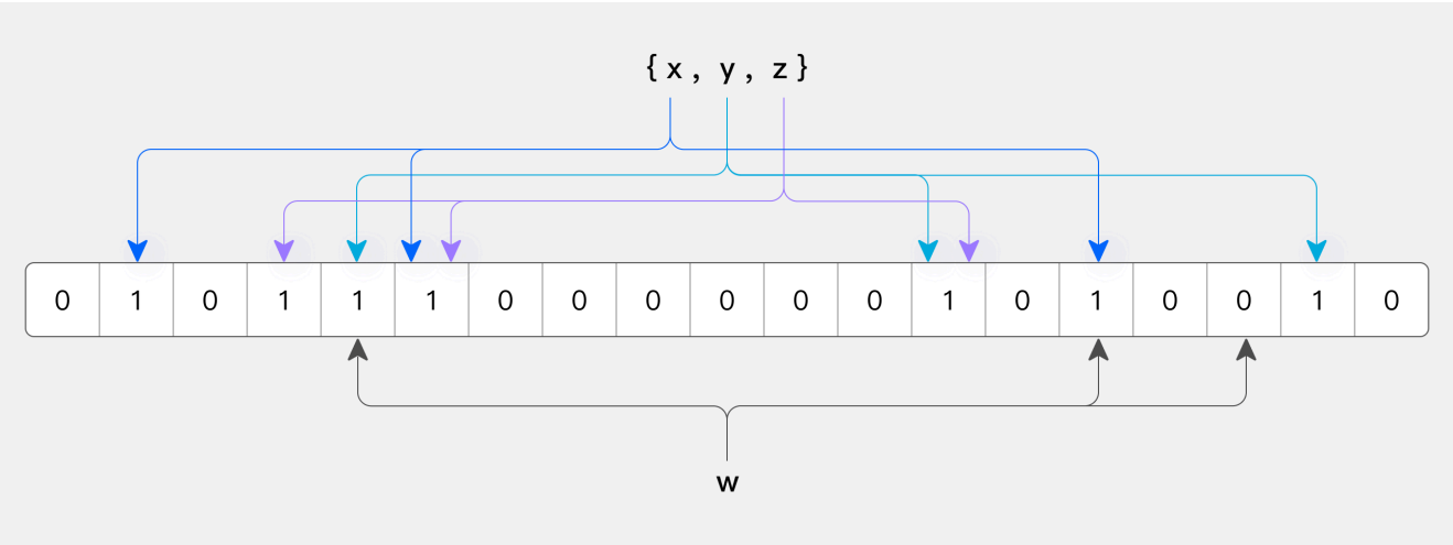
Bloom_filter.svg
