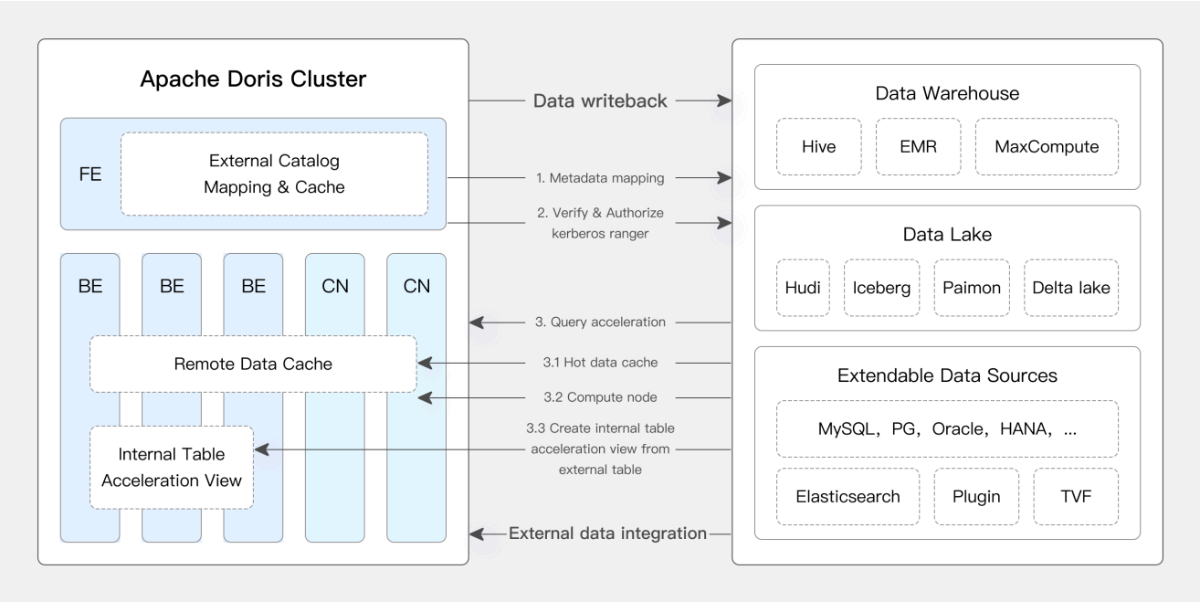
基于 Doris 的湖仓一体架构
