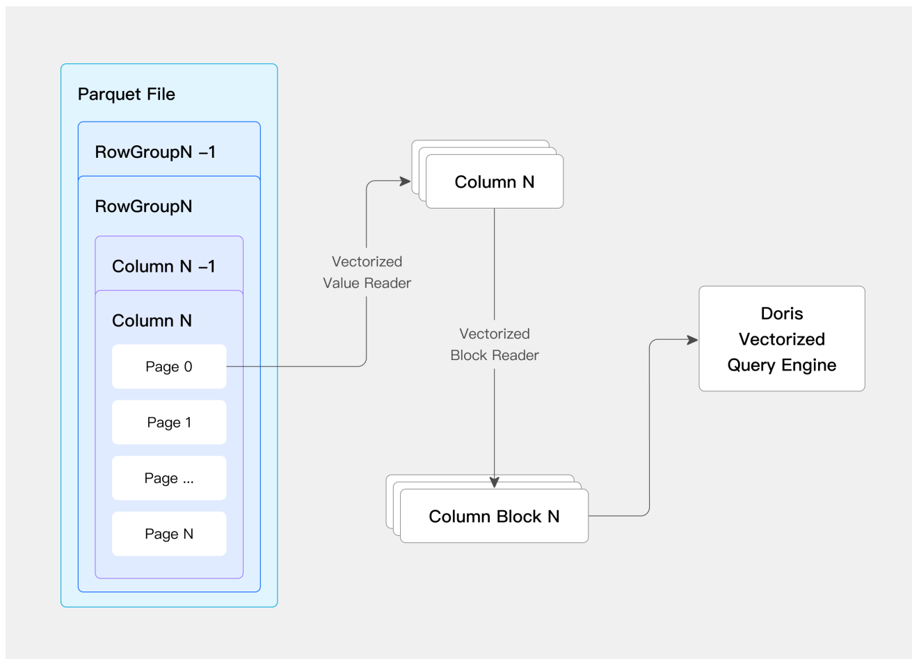
向量化读取数据
